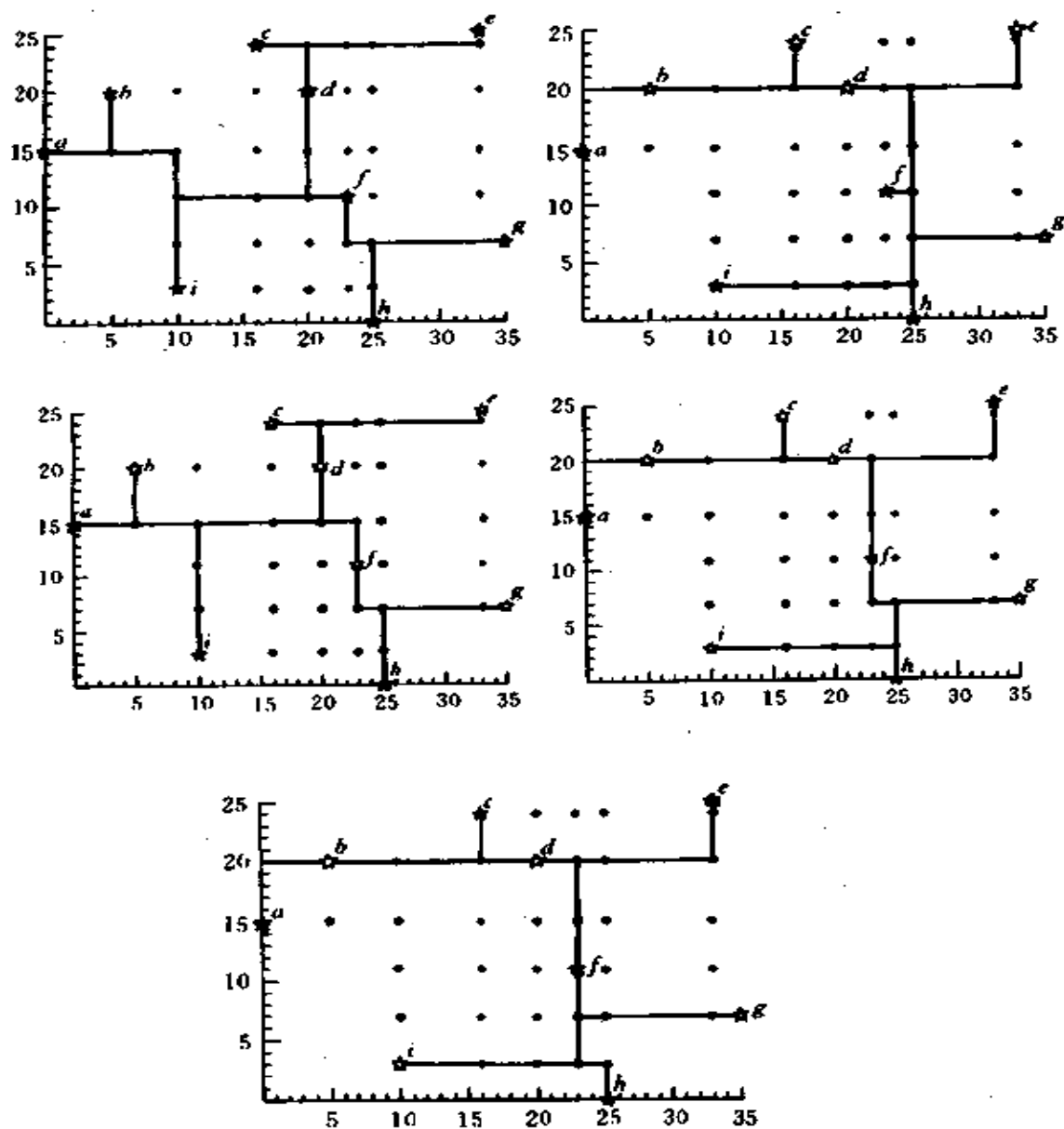
图 23-7 5 个费用最少的 Steiner 树
